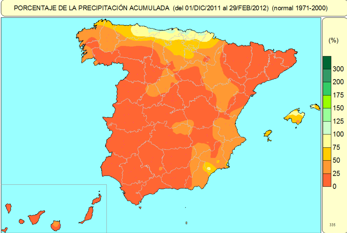
Mapa de porcentaje de las precipitaciones acumuladas en el trimestre invernal de 2011-2012 sobre el valor medio normal.
